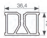
wymiary niskiego legara aluminiowego (mm)
