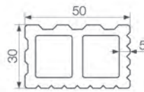
wymiary legara (mm)
